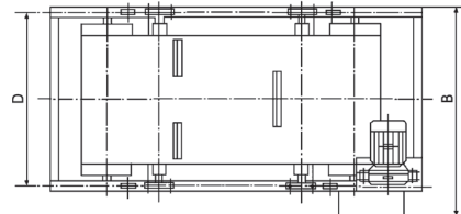
外形尺寸图
